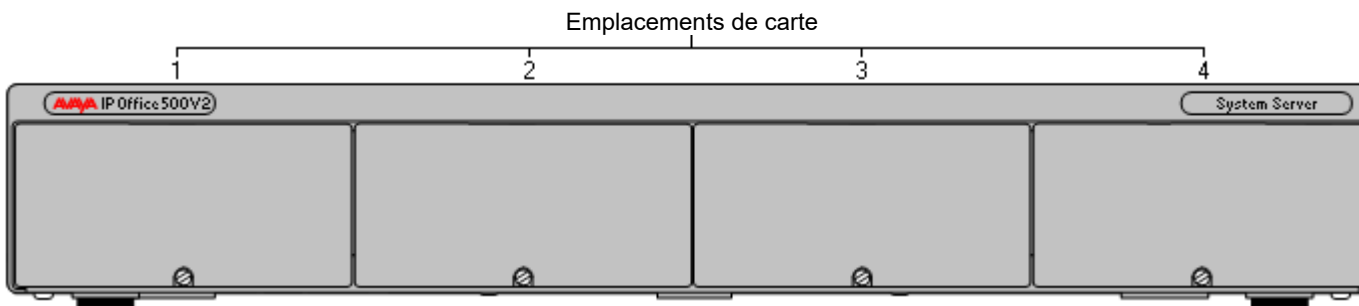
Illustration 5 : IP500 V2 - face avant
