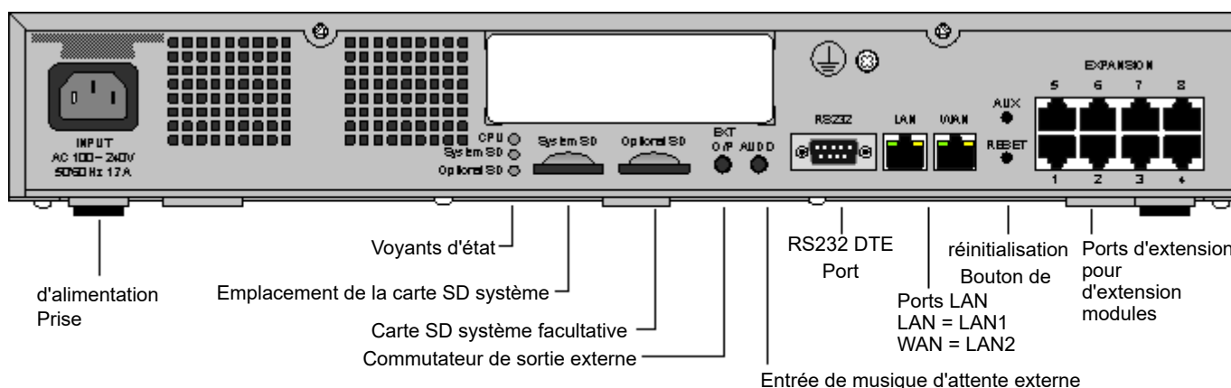
Illustration 6 : IP500 V2 - vue arrière
