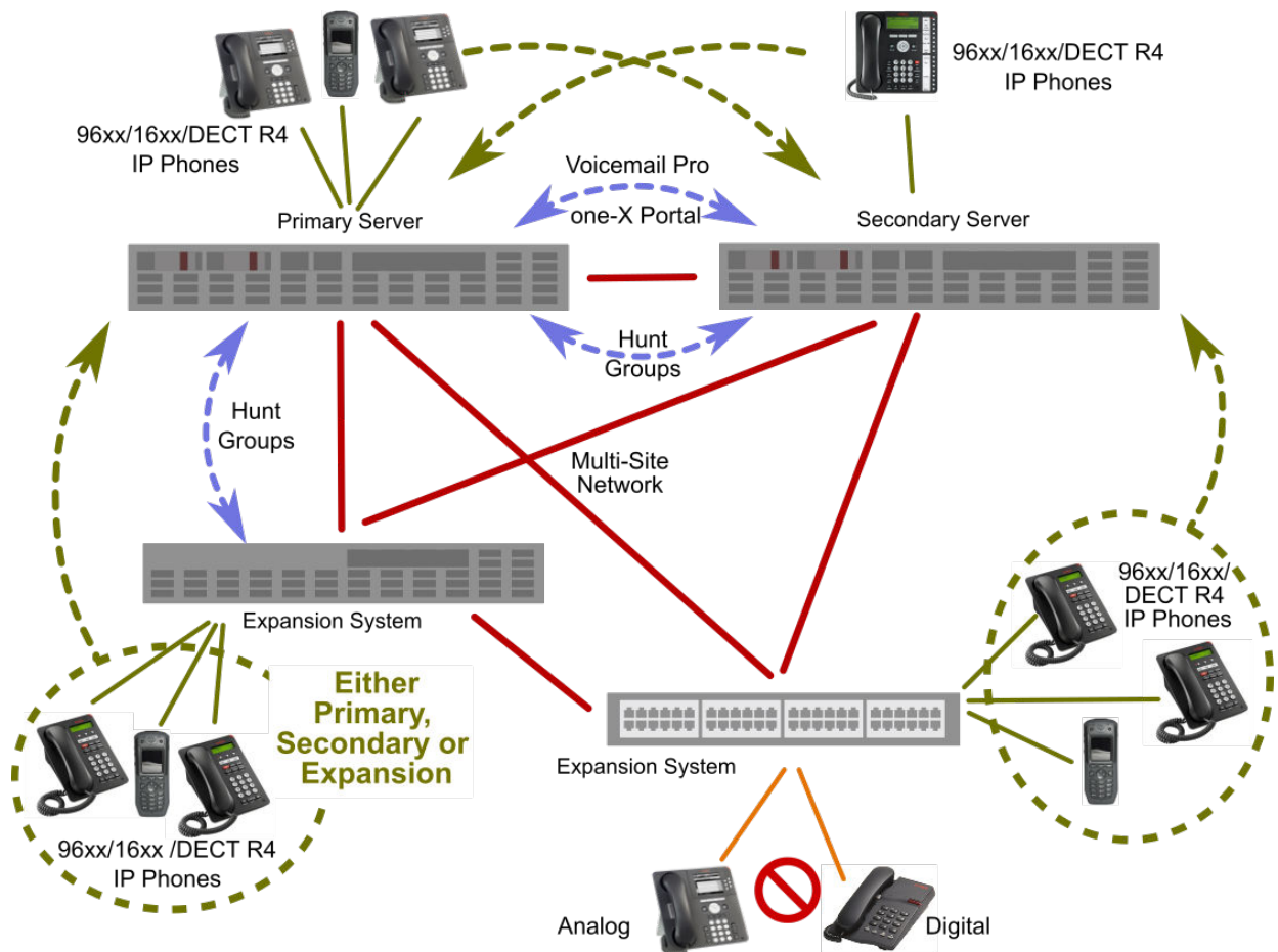
Illustration 2 : Architecture de résilience
