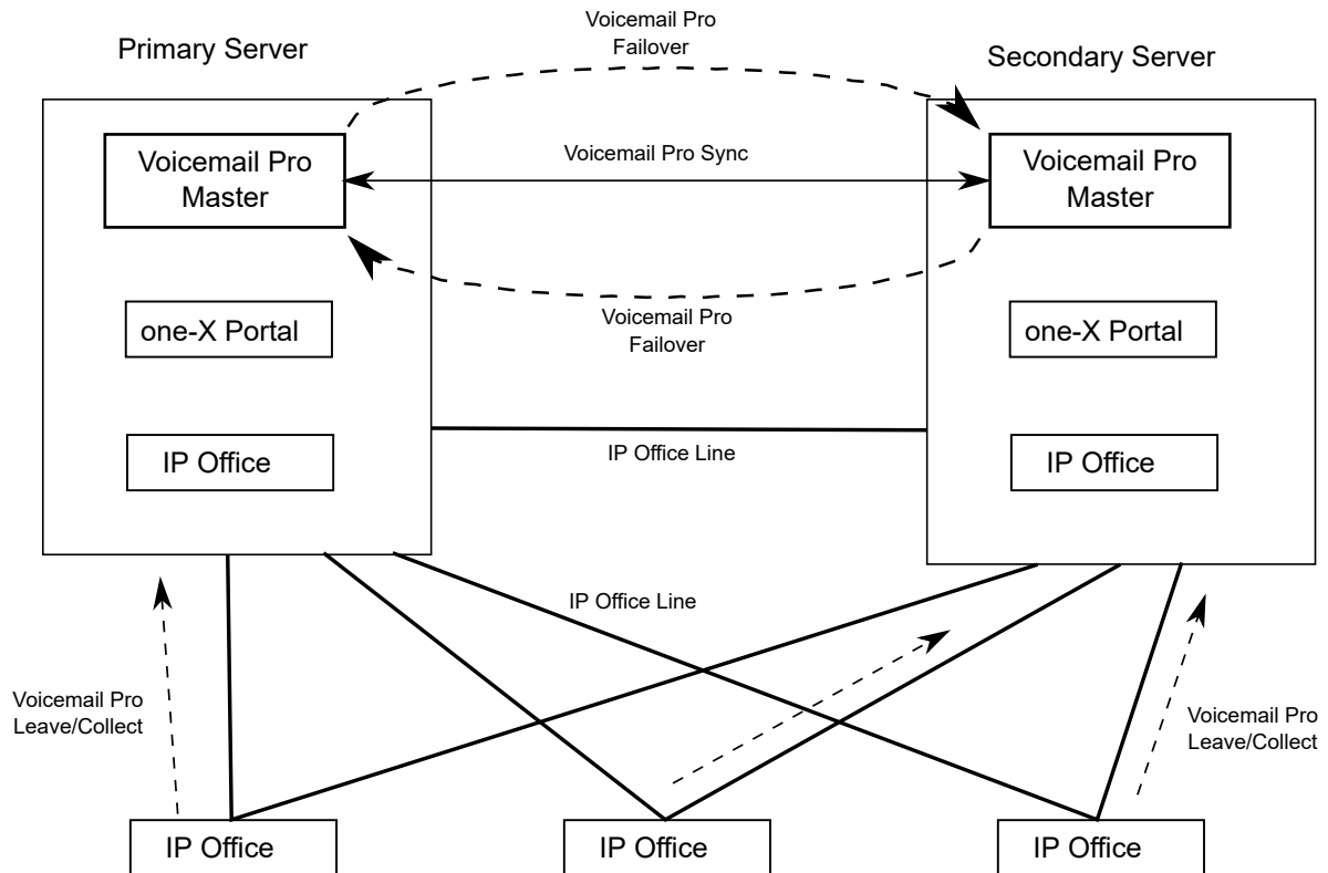
Illustration 4 : Deux serveurs Voicemail Pro actifs
